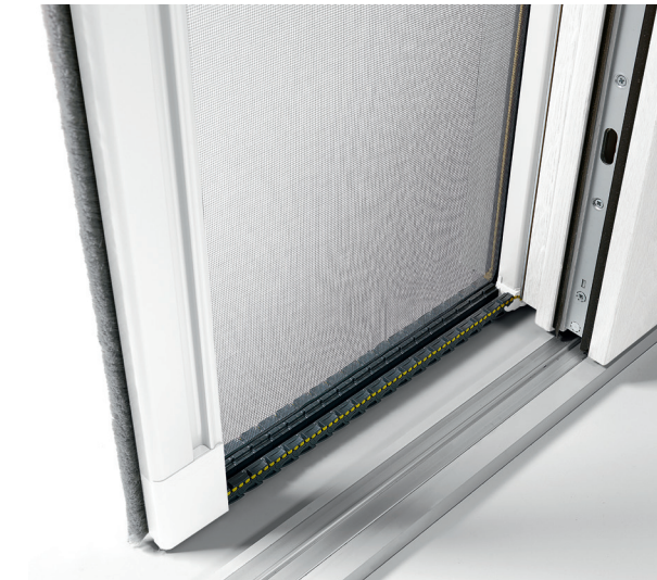
Particolare zanzariera miniscenica a scomparsa. Close up: retractable Miniscenica insect screen.
